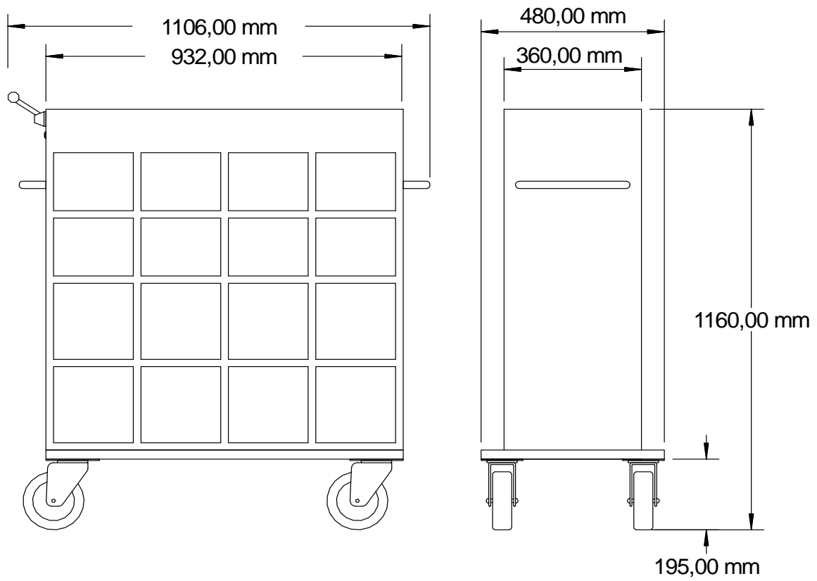
Cash and mini tipbox trolley ;8+8 boxes
