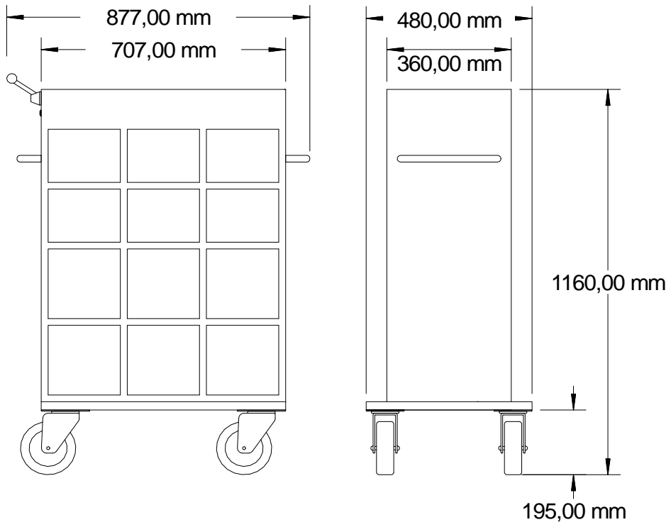
Cash and mini tipbox trolley ; 6+6 boxes
